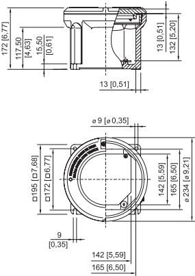
Boîtier taille 3 sans hublot
