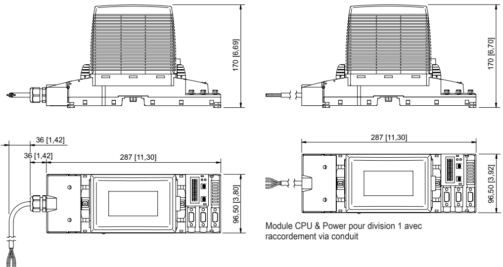
Module CPU & Power pour zone 1 avec raccordement via connecteur précâblé
