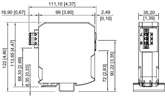
Plan d'encombrement (toutes les dimensions sont en mm [pouces]) – sous réserve de modifications
