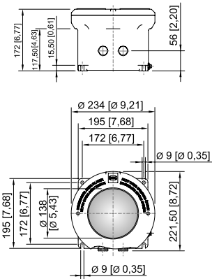
Boîtier taille 3 avec hublot
