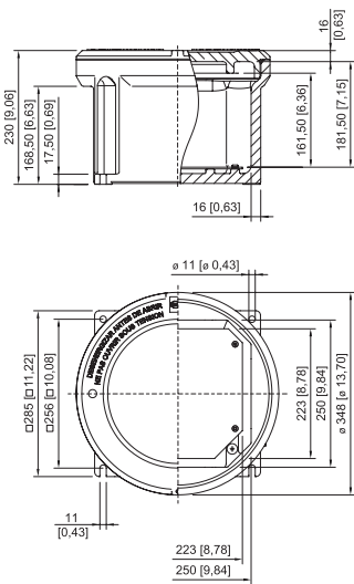
Boîtier taille 5 sans hublot
