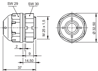
Plan d'encombrement (toutes les dimensions sont en mm [pouces]) – sous réserve de modifications
