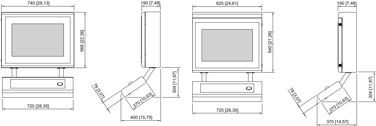
Plan d'encombrement (toutes les dimensions sont en mm [pouces]) – sous réserve de modifications
