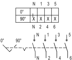
Schéma de fonctionnement 8544/1-4 and 8549/1-4
