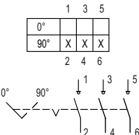
Schéma de fonctionnement 8544/1-3 and 8549/1-3
