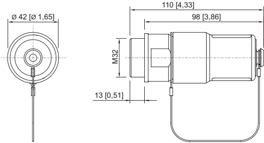
8595/1 Prise de courant à bride Ex e
