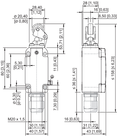
Levier à galet 8074/2--WH-40
