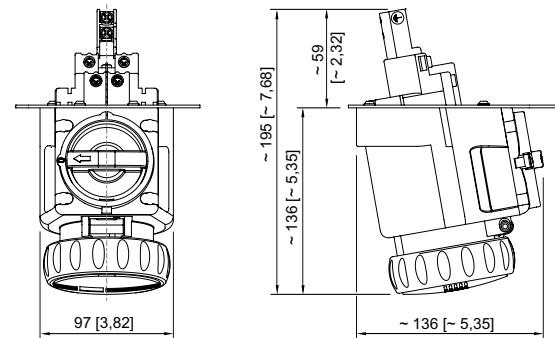
Prise de courant à bride 5 pôles Position horaire 9 h, 10 h, 11 h
