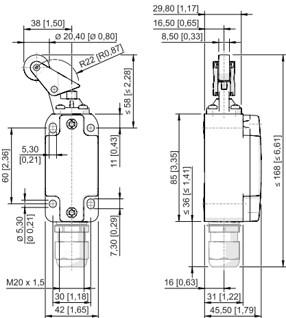
Roller lever 8070/2-WPH-U60
