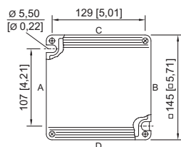
8118/.3. Enclosure SZ 3
