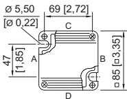
8118/.1. Enclosure SZ 1
