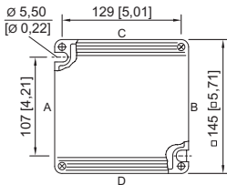
8118/.3. Enclosure SZ 3
