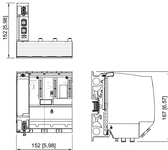
CPU 模块 9442/32 + 底座 9496/32-04-00
