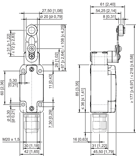
Schwenkhebel 8070/2-3-DS-U60
