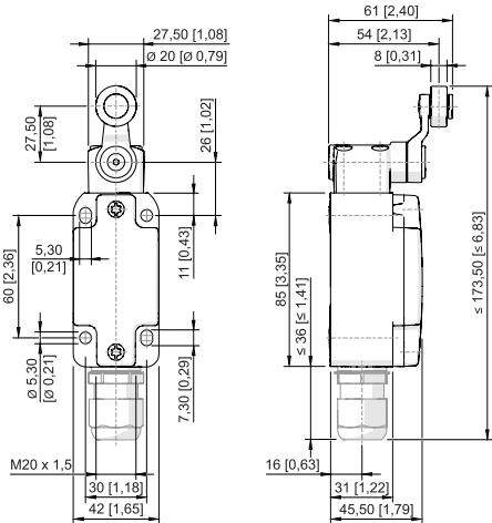
Schwenkebel 8070/2--D-U60
