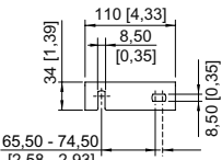
Wandbefestigungswinkel montiert in Montageschiene
