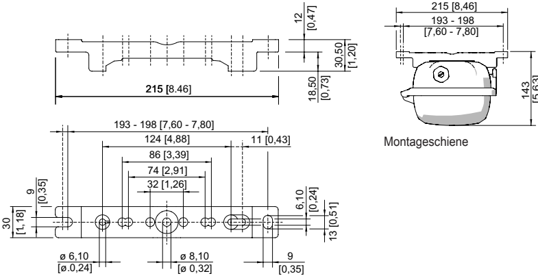
Montageschiene
