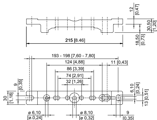
Montageschiene
