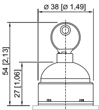
8003/...-008 Schlüsselschalter
