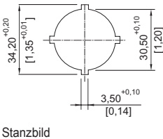
Stanzbild
