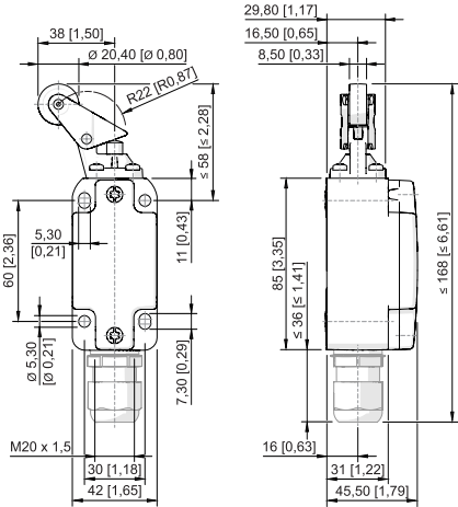
Rollenhebel 8070/2-3-WPH-U60
