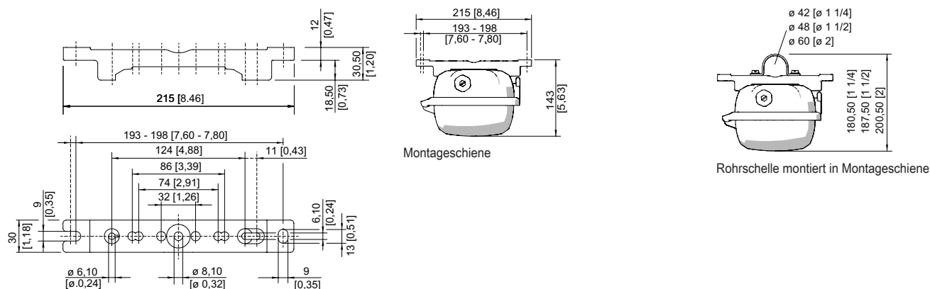
Montageschiene
