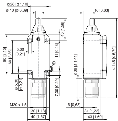
Kuppenstößel 8074/2-W-40
