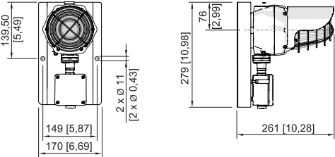
Maßzeichnung (alle Maße in mm [Zoll]) – Änderungen vorbehalten
