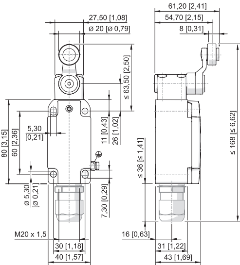
Schwenkhebel 8074/2--D-40
