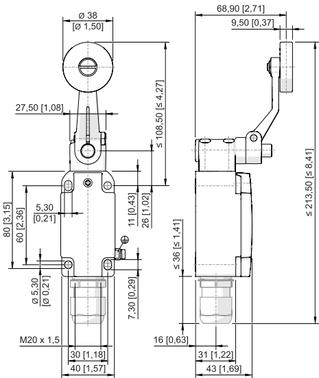
Stangenhebel 8074/2-3-DL-40
