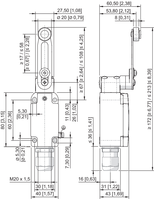
Schwenkhebel 8074/2-1-DS-40
