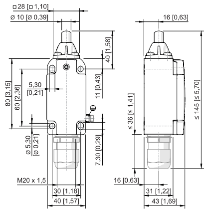
Kuppenstoßel 8074/2-1-W-40
