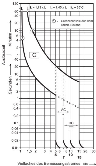
Auslösecharakteristik C
