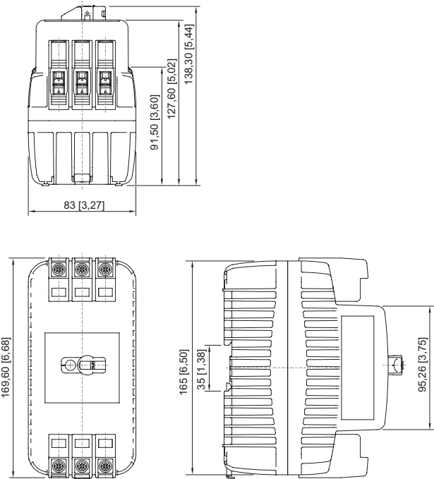
8530/1; 3 Teilungseinheiten
