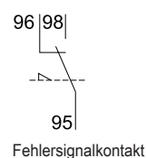
Fehlersignalkontakt
