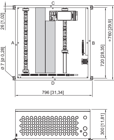
1 x BusRail für 10 Steckplätze
