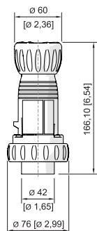
Stecker Kleinspannung
