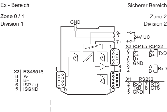
Anschlussplan 9185/11
