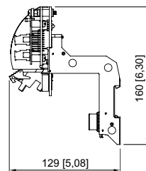
9419/04R bus-Träger für 4 Feldbus-Segmente
