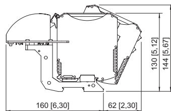
9419 bus-Träger mit Modulen
