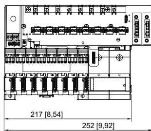
9419/08F bus-Träger für 8 Feldbus-Segmente
