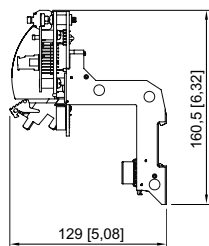
9419/08F bus-Träger für 8 Feldbus-Segmente
