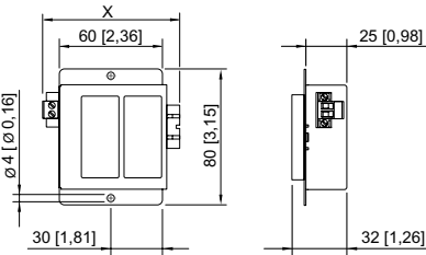
Maßzeichnung (alle Maße in mm [Zoll]) – Änderungen vorbehalten
