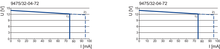
Ausgangskennlinie 9475/32-04-72
