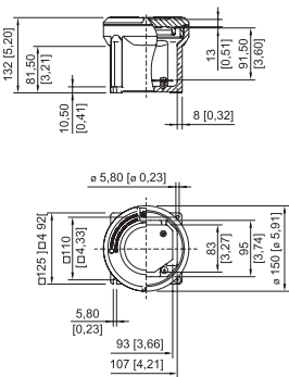
Gehäuse Größe 1 ohne Schauglas
