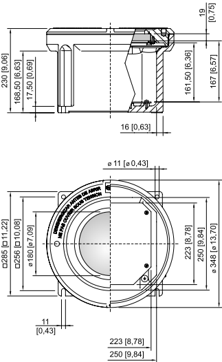
Gehäuse Größe 5 mit Schauglas
