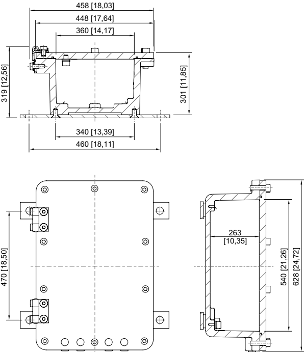
Maßzeichnung (alle Maße in mm [Zoll]) – Änderungen vorbehalten
