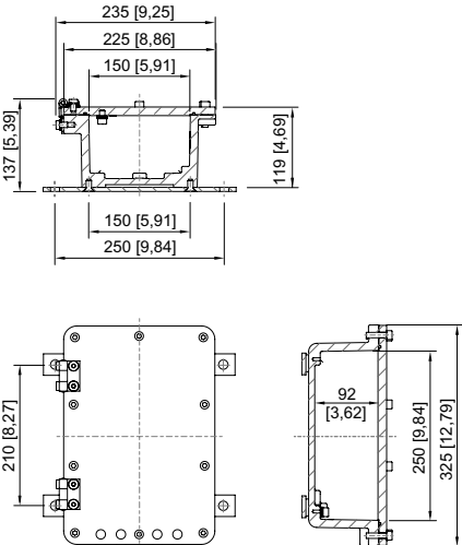
Gehäusegröße 1
