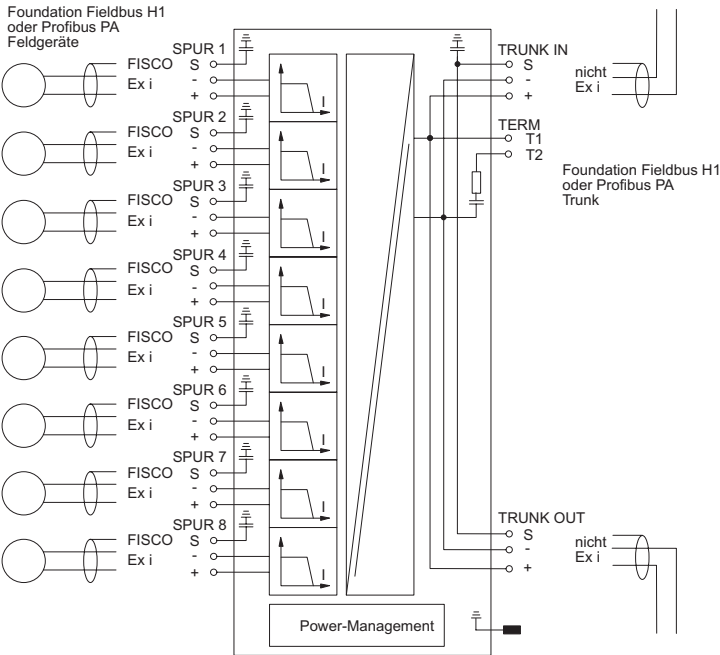
Anschlussplan 9411/2.
