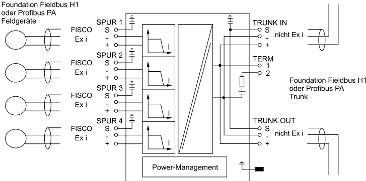
Anschlussplan 9411/2.
