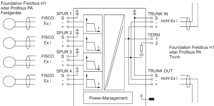
Anschlussplan 9411/2.
