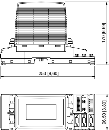
CPU & Power Modul für Zone 1 mit Anschluss über Ex e Klemmen
