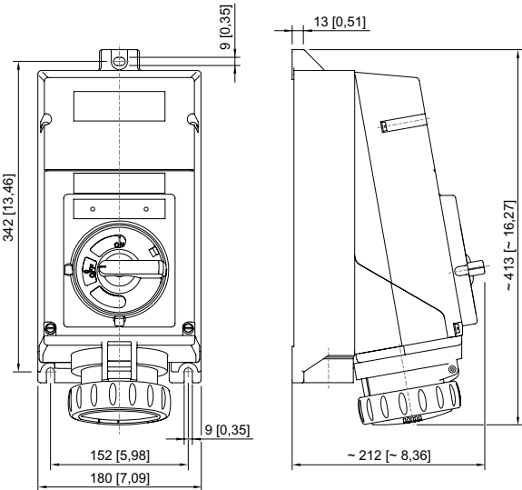
Wandsteckdose
