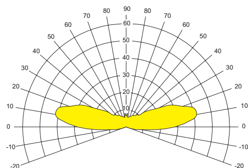
Lichtverteilungskurve
