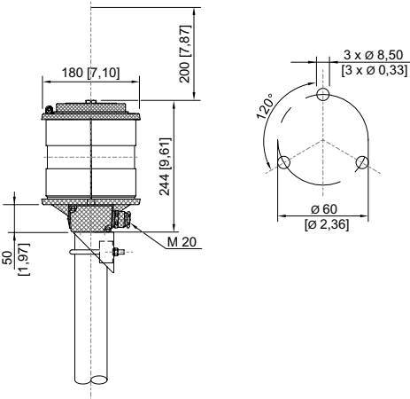
TEF 2850 Rundum-Navigationsleuchte
